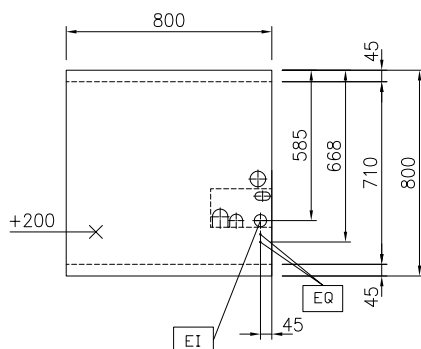
Boven aanzicht
